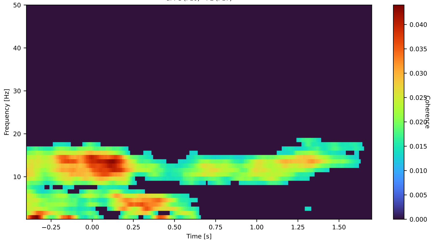
dPFC (F10) - PE (P17)
